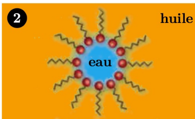
Goutte d'eau encapsulée dans l'huile
