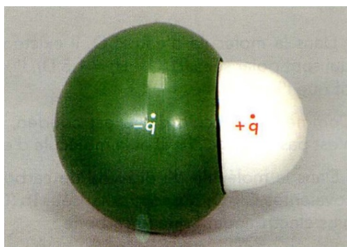
FIG. 2 – Modèle moléculaire du chlorure d'hydrogène.
