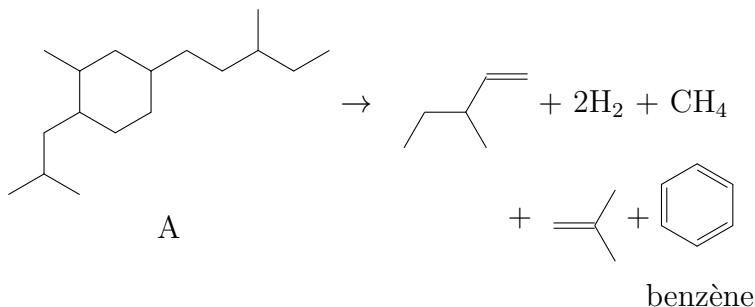
FIG. 2 – Exemple de réaction de craquage.
